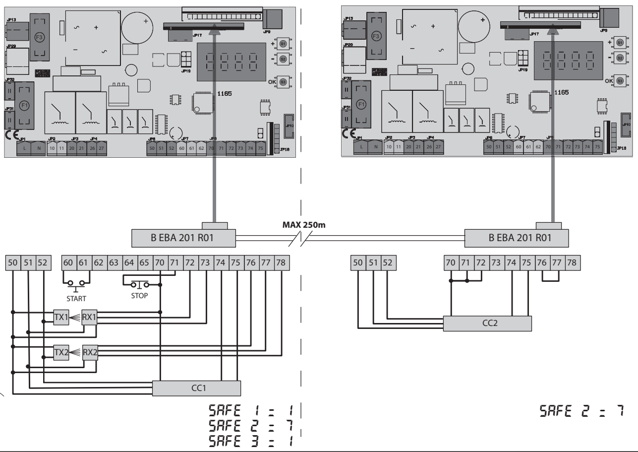
ESEMPIO APPLICAZIONE ANTE CONTRAPPOSTE CON 2 PHOT E 2 BAR - SAMPLE APPLICATION WITH OPPOSITE LEAVES WITH 2 PHOT AND 2 BAR - EXEMPLE D'APPLICATION VANTAUX OPPOSÉS AVEC 2 PHOT ET 2 BAR - ANWENDUNGSBEISPIEL EINANDER ENTGEGENGESETZTE TORFLÜGEL MIT 2 PHOT UND 2 BAR - VOORBEELD TOEPASSING TEGENOVERGESTELDE VLEUGELS MET 2 PHOT EN 2 BAR
